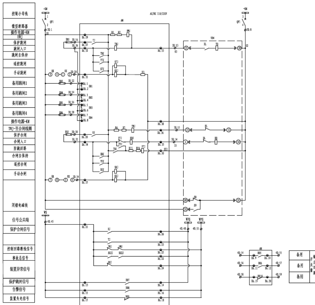
图 6.35 AM5SE-MD 二次原理图（三）
