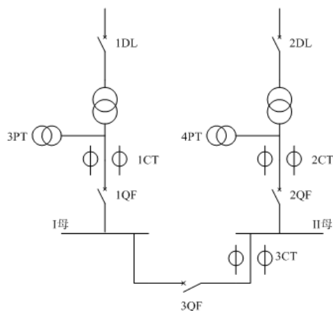
图 4.5.3 两进线一母联系统采集两路进线电压一次图
