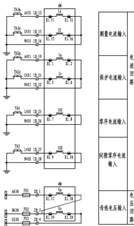
图 8.17 2PT 2CT 接线方法
