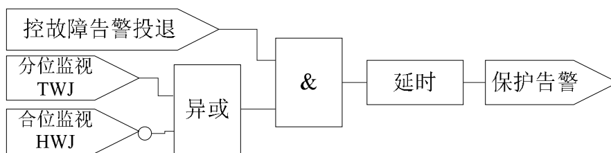
图 2.7 控制回路断线告警逻辑
