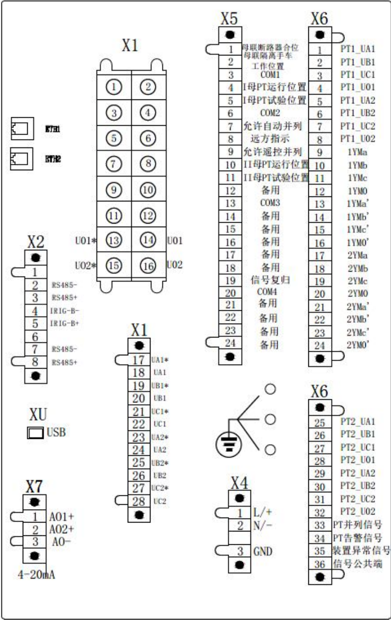
图 9.13 AM5SE-UB 电气接线图
