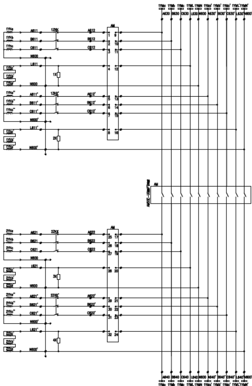
图 9.17 AM5SE-UB 二次原理图（三）
