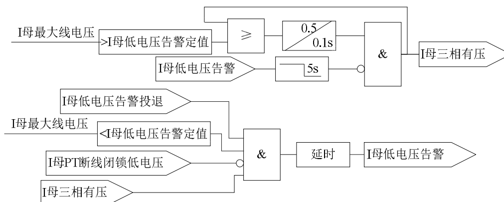
图 9.5 I 母 PT 低电压告警逻辑
