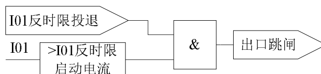
图 2.4 I01 反时限过流保护逻辑
