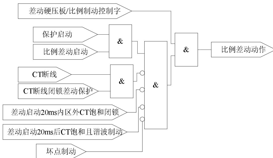
图 6.1 比例制动差动保护动作逻辑
