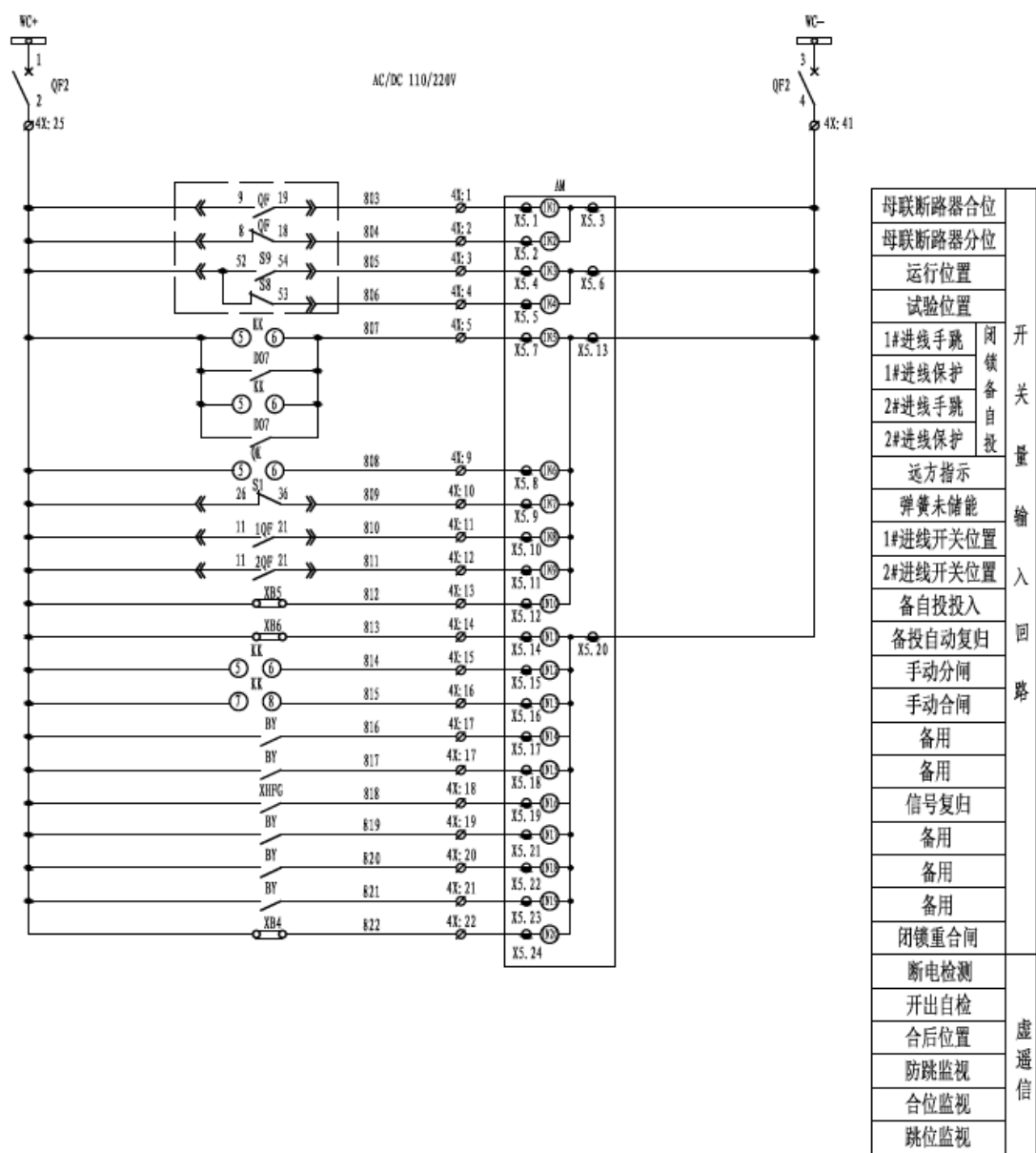
图 4.14 AM5SE-B 备自投二次原理图（二）
