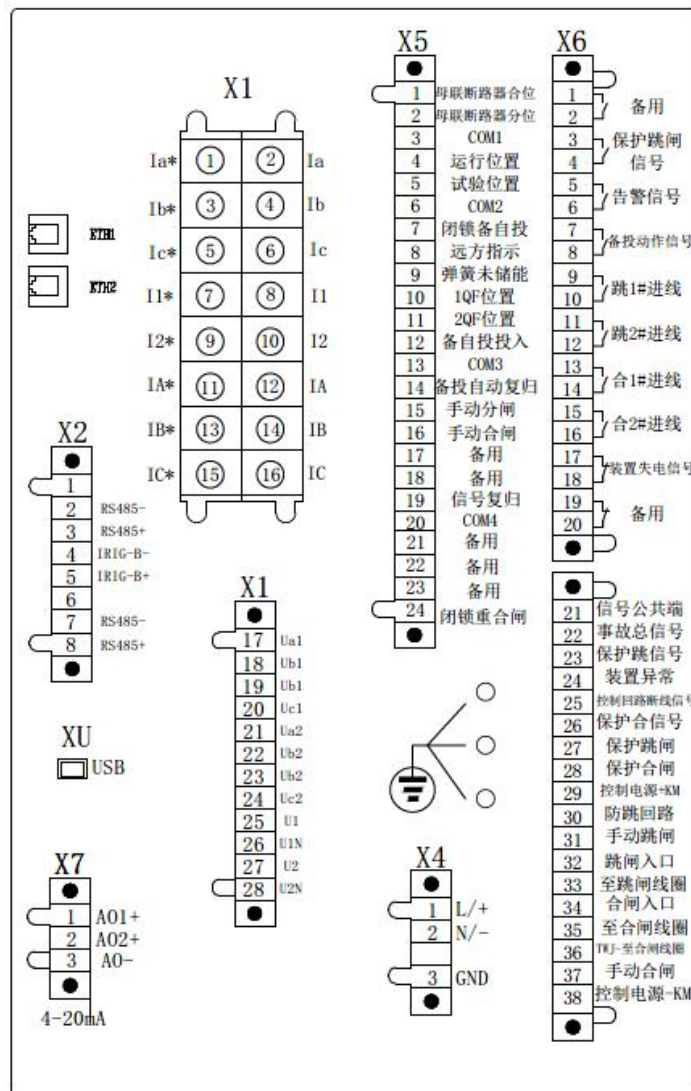
图 4.12 AM5SE-B 电气接线图
