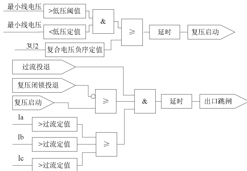
图 2.1 三段式过流保护逻辑
