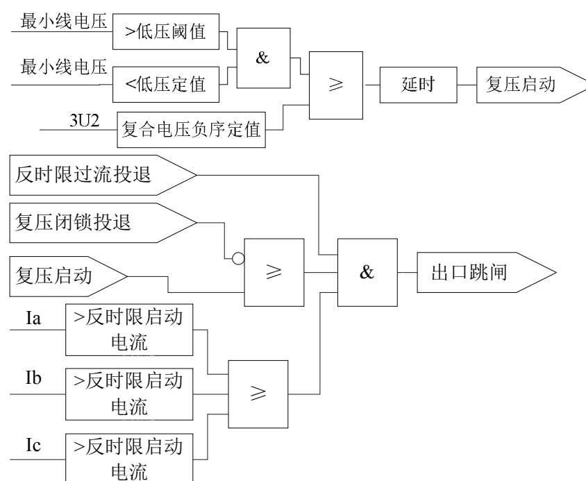
图 4.3 反时限过流保护逻辑
