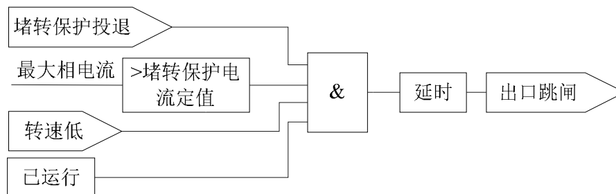
图 3.9 堵转保护逻辑
