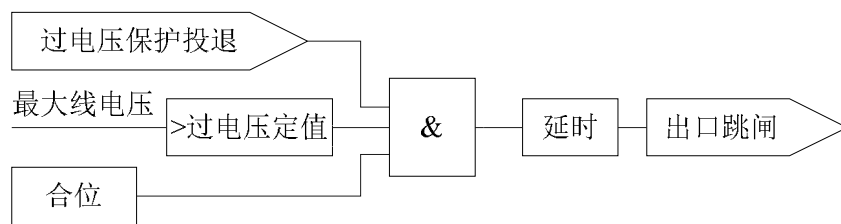
图 5.5 过电压保护逻辑
