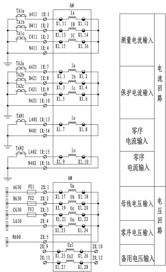
图 3.24 AM5SE-M 二次原理图（一）
