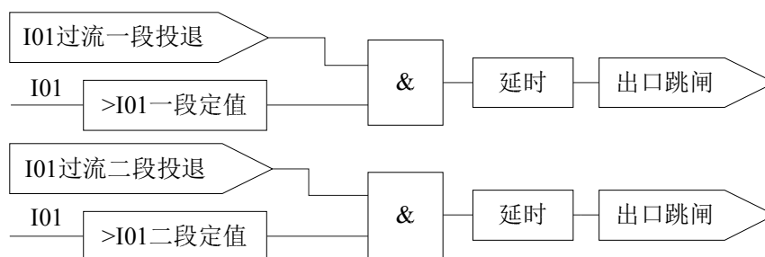
图 3.6 两段式零序过流保护逻辑
