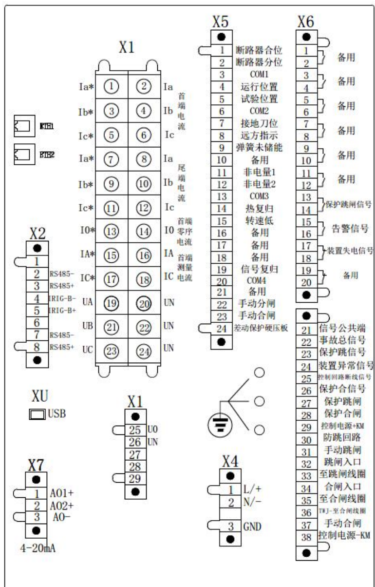
图 6.31 AM5SE-MD 电气接线图
