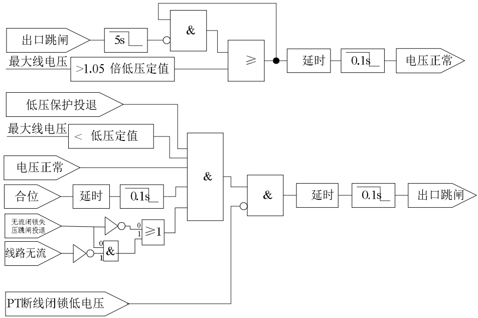
图 3.12 低电压保护逻辑
