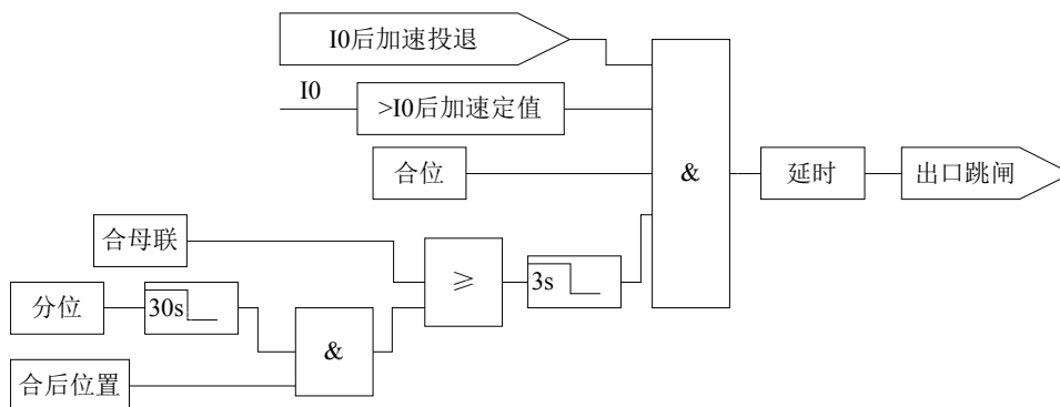
图 4.11 零序后加速过流保护逻辑
