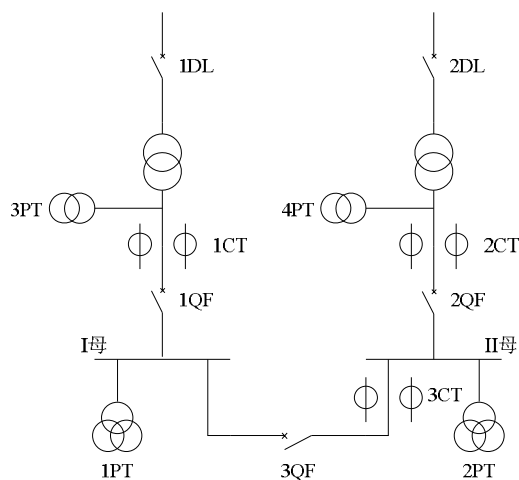
图 4.5.1 两进线一母联系统采集进线母线 6 路电压一次图
