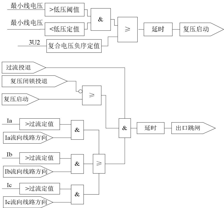
图 4.2 三段式过流保护逻辑
