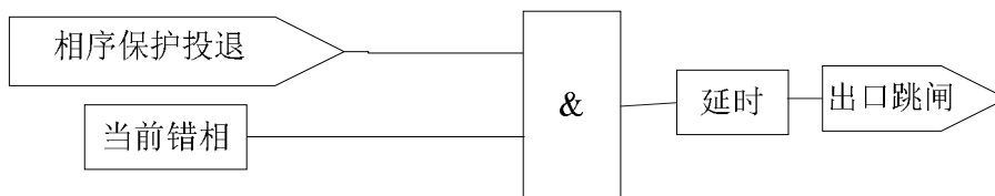
图 3.19 相序保护逻辑
