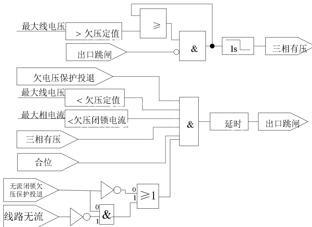
图 5.4 欠电压保护逻辑
