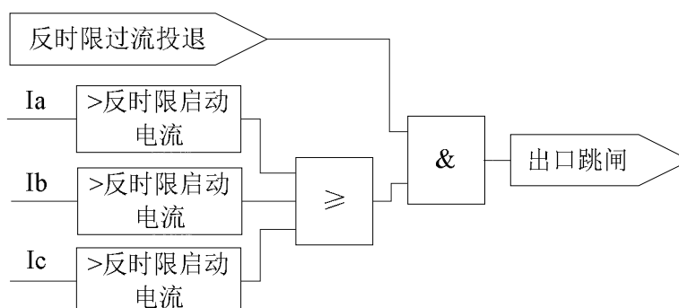
图 5.2 反时限过流保护逻辑
