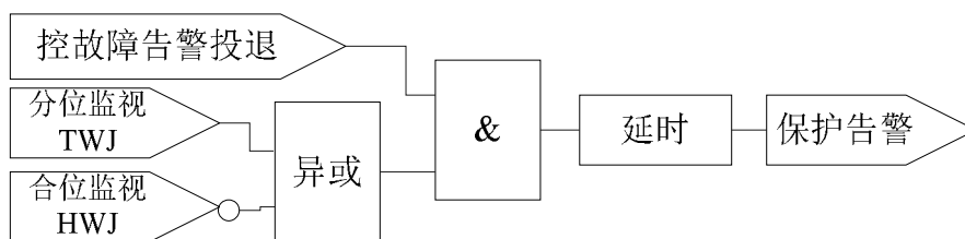
图 6.30 控制回路断线告警逻辑
