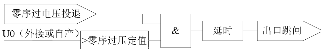
图 5.6 零序过电压保护逻辑
