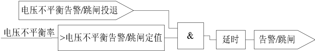
图 6.24 电压不平衡保护逻辑
