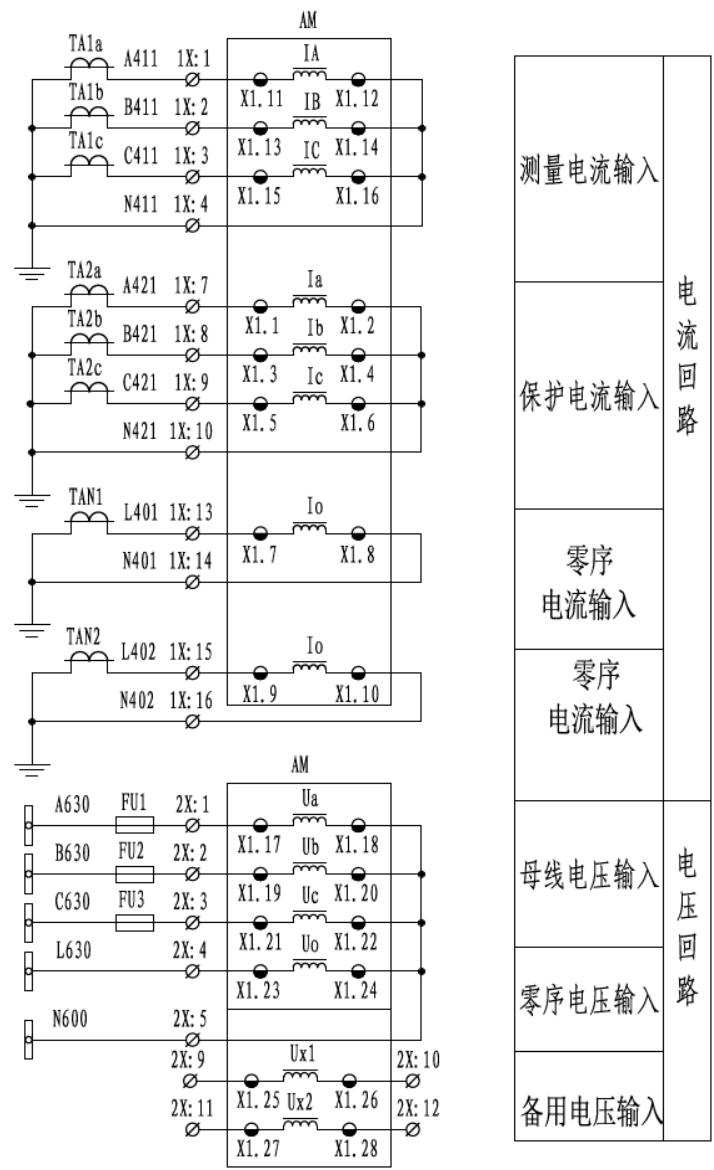
图 1.17 AM5SE-F 二次原理图（一）
