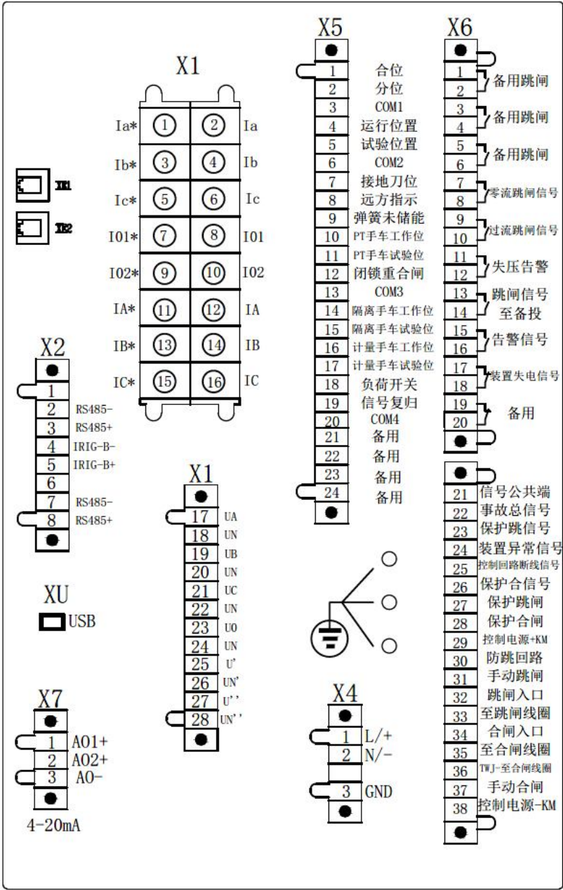
图 1.15 AM5SE-F 电气接线图
