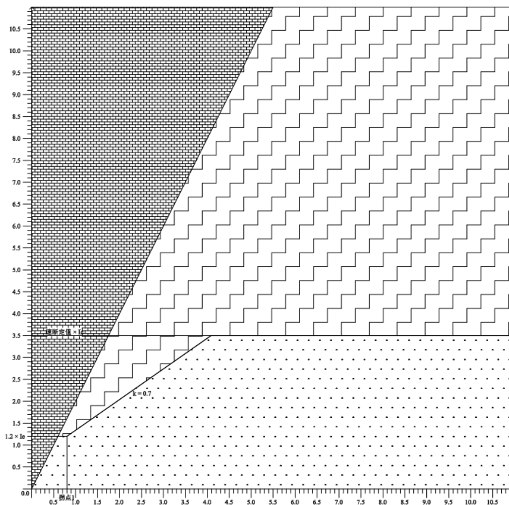
图 7.2 比例制动差动保护曲线一
