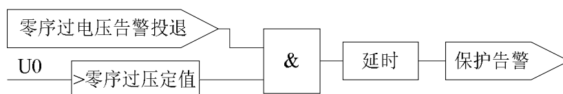
图 3.16 零序过压告警逻辑
