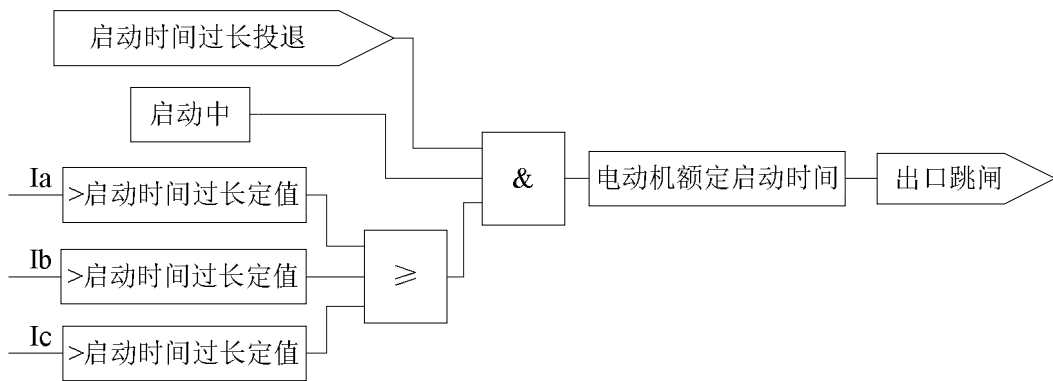
图 3.11 启动时间过长保护逻辑
