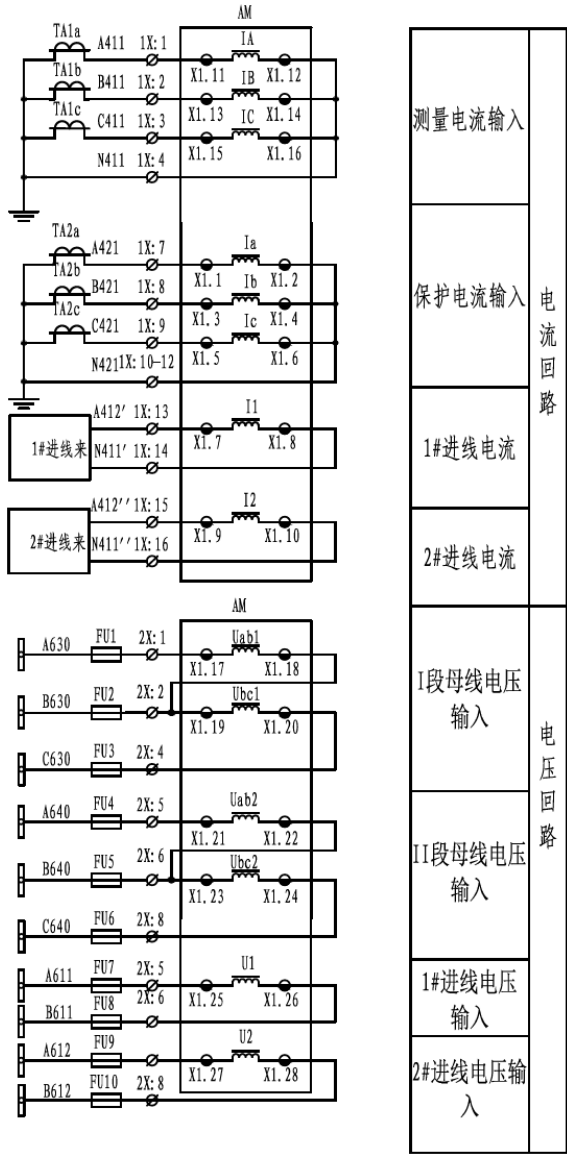
图 4.13 AM5SE-B 备自投二次原理图（一）
