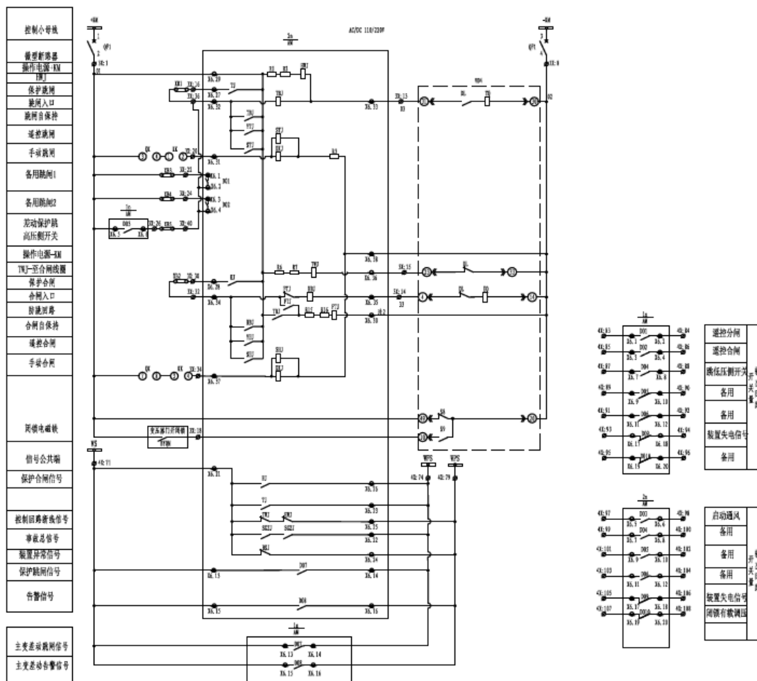
图 8.20 AM5SE-TB 二次原理图 (三)
