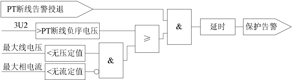
图 5.10 PT 断线告警逻辑
