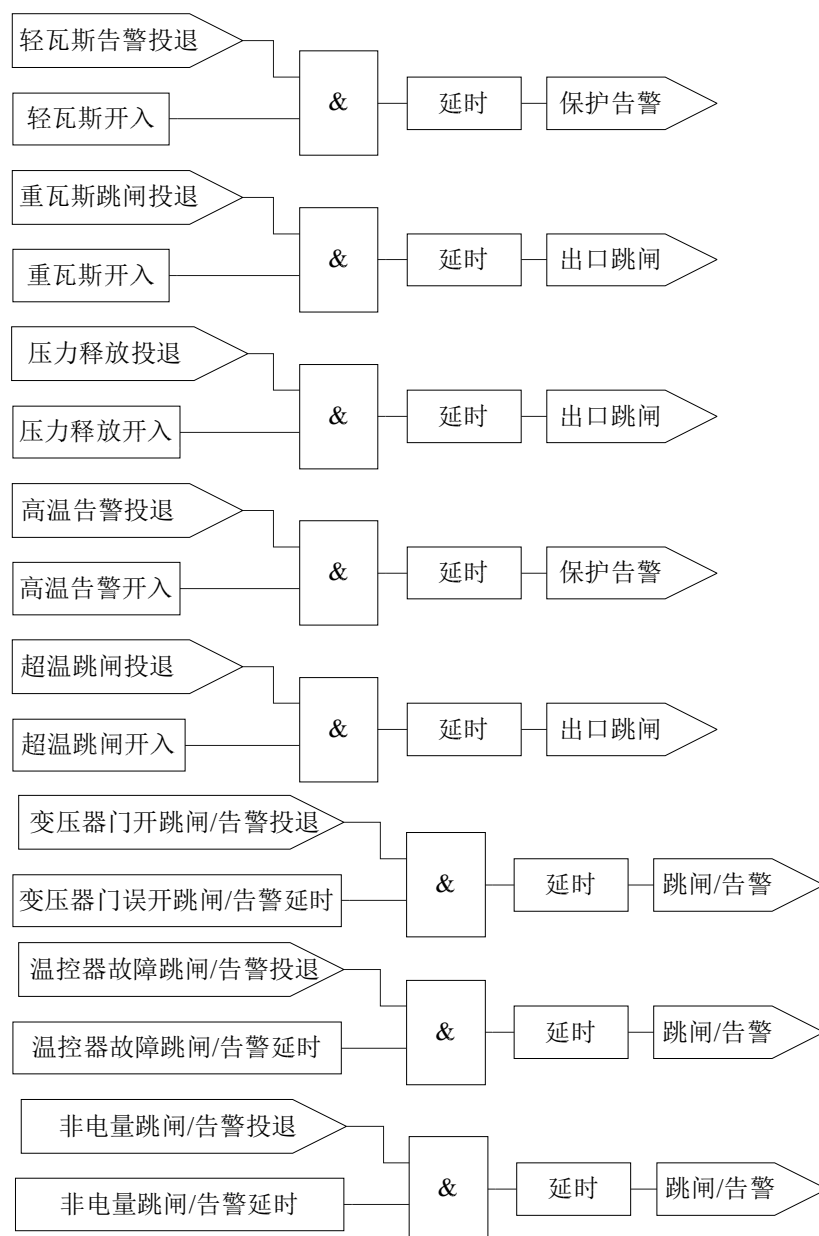
图 8.9 非电量保护逻辑
