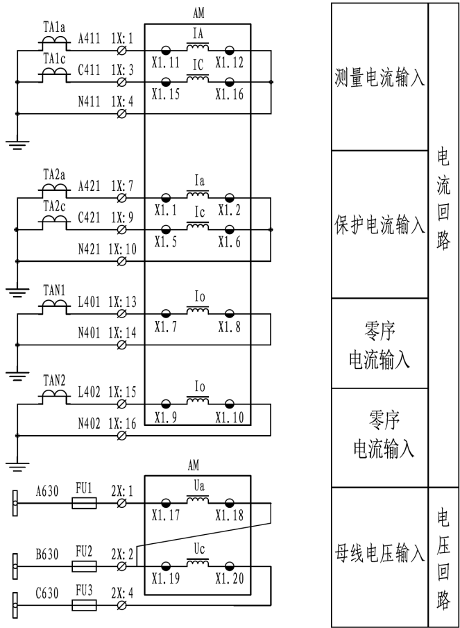
图 3.23 2PT 2CT 接线方法
