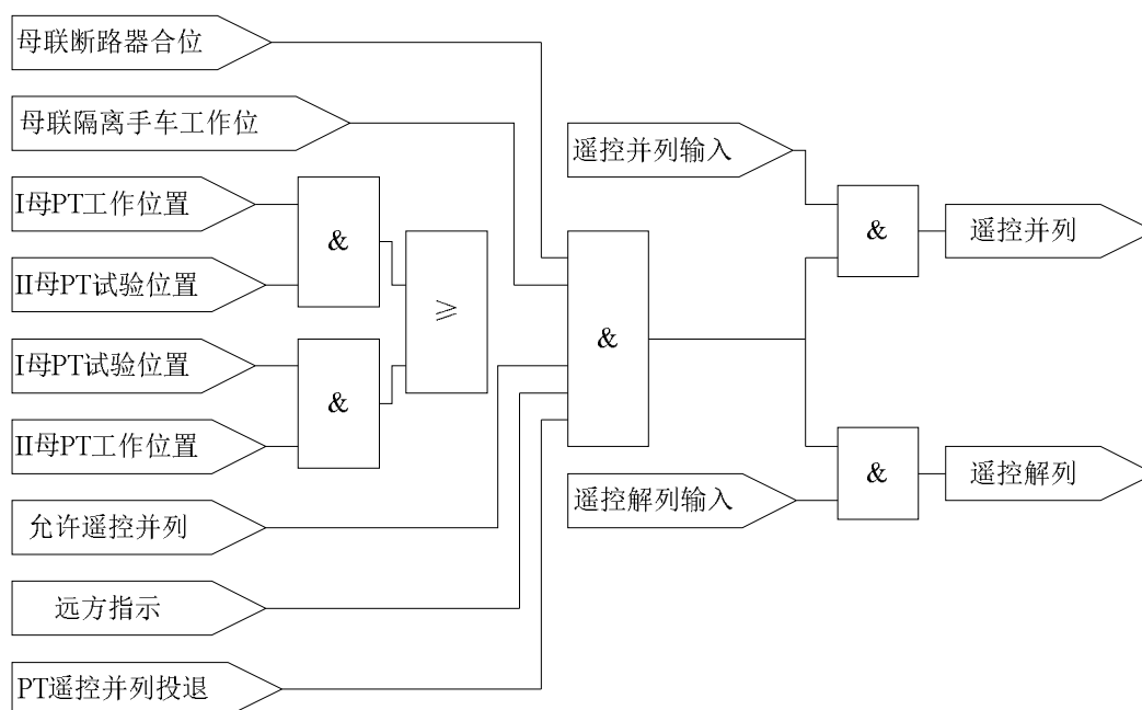
图 9.4 PT 遥控并列解列逻辑
