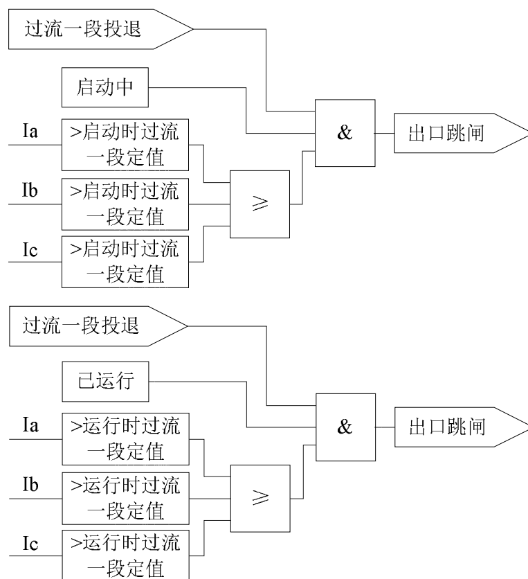
图 3.1 过流一段保护逻辑
