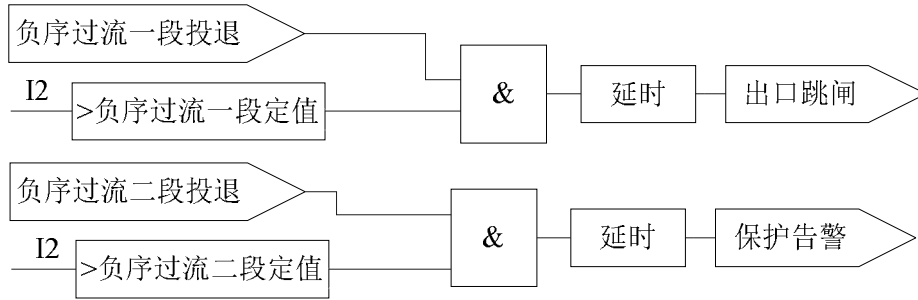
图 3.4 两段式负序过流保护逻辑
