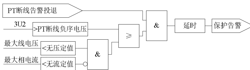
图 3.14 PT 断线告警逻辑
