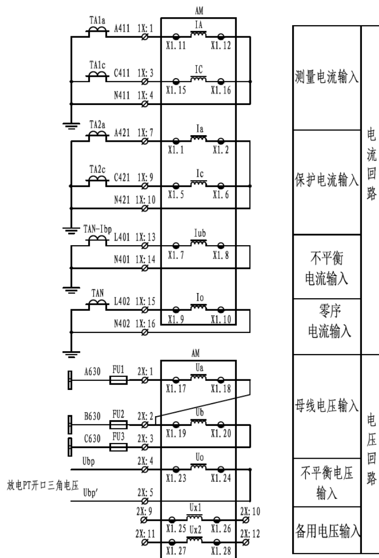
图 5.13 2PT 2CT 接线方法
