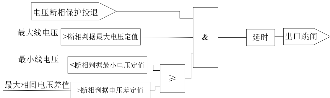
图 3.20 电压断相保护逻辑
