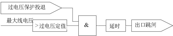
图 3.21 过电压保护逻辑
