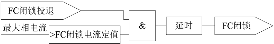
图 1.10 FC 回路配合的过流闭锁功能逻辑
