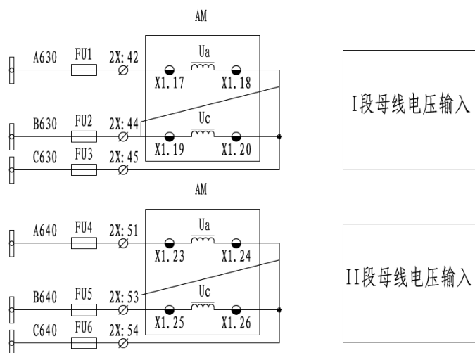
图 9.14 2PT 接线方法
