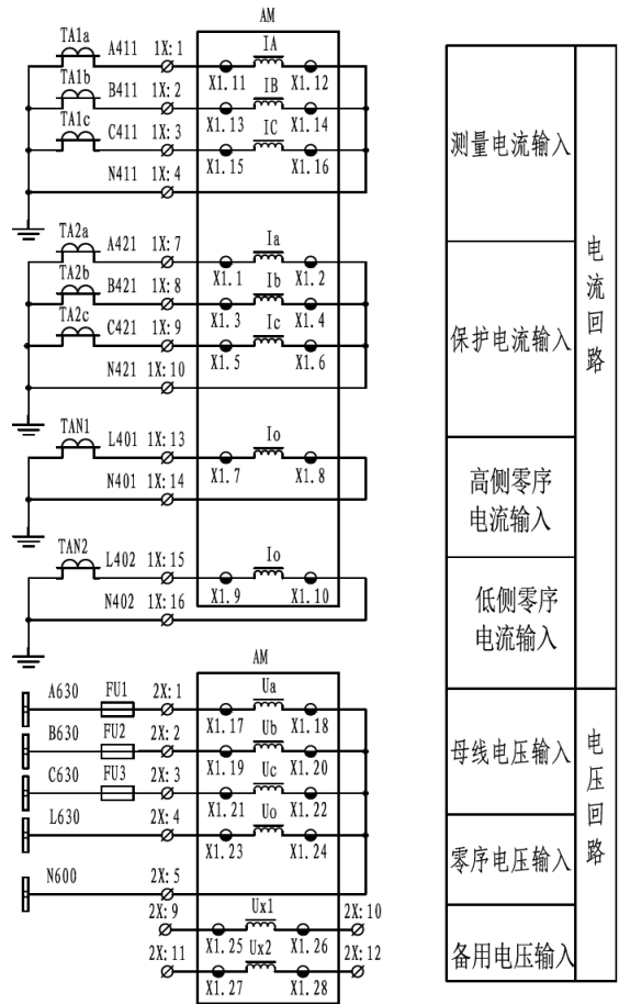
图 2.12 AM5SE-T 二次原理图（一）
