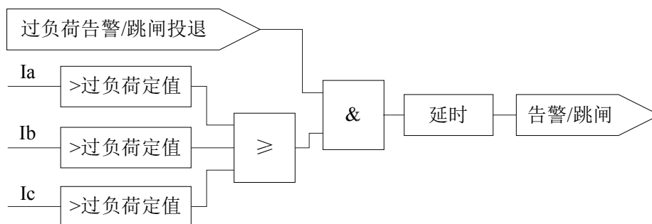
图 1.6 过负荷保护逻辑
