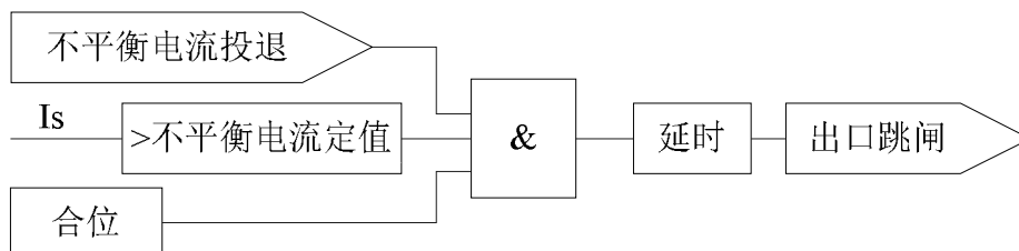
图 5.8 不平衡电流保护逻辑
