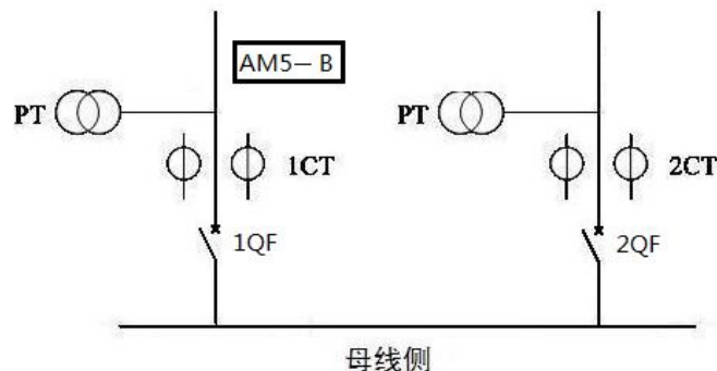
图 4.5.4 两进线无母联系统采集两路进线电压一次图
