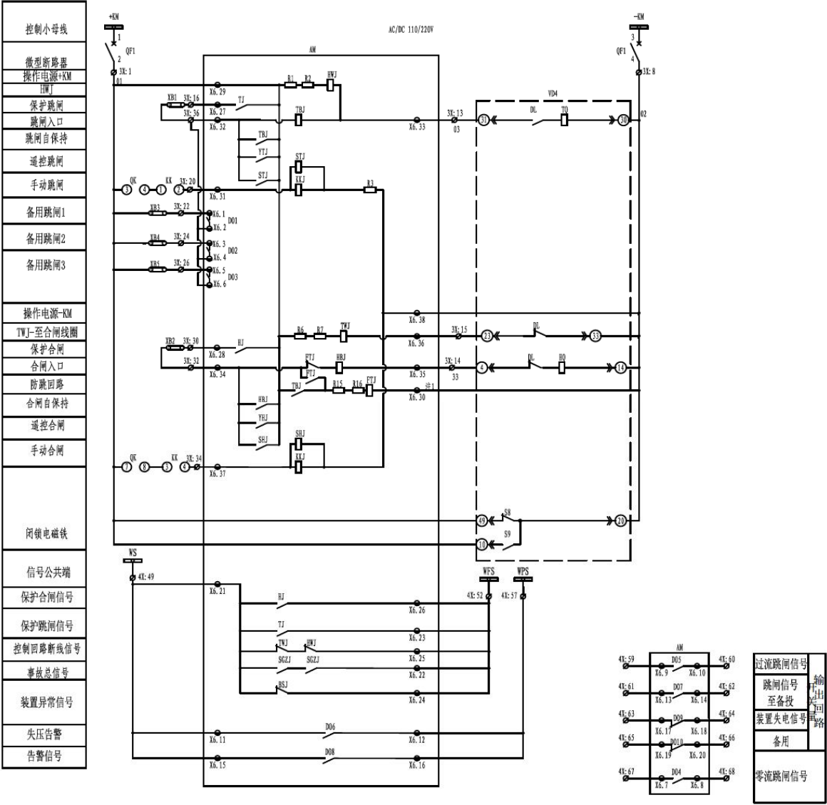
图 1.19 AM5SE-F 二次原理图 (三)
