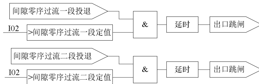
图 8.10 两段式间隙零序过流保护逻辑
