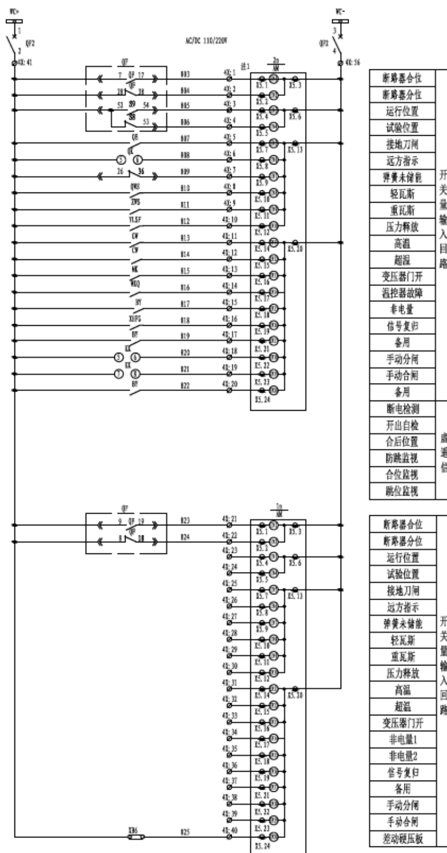
图 8.19 AM5SE-TB 二次原理图（二）
