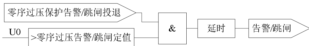
图 6.21 零序过压保护逻辑
