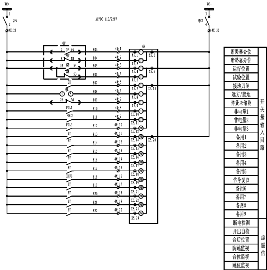
图 5.15 AM5SE-C 二次原理图（二）
