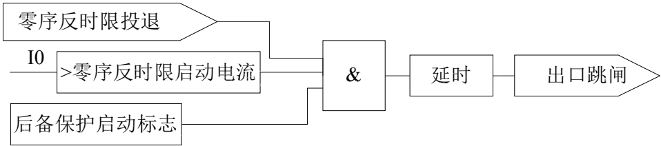
图 6.10 零序反时限过流保护逻辑
