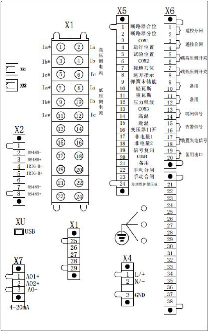
图 7.5 AM5SE-D2 电气接线图
