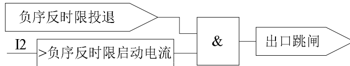
图 3.5 负序反时限过流保护逻辑
