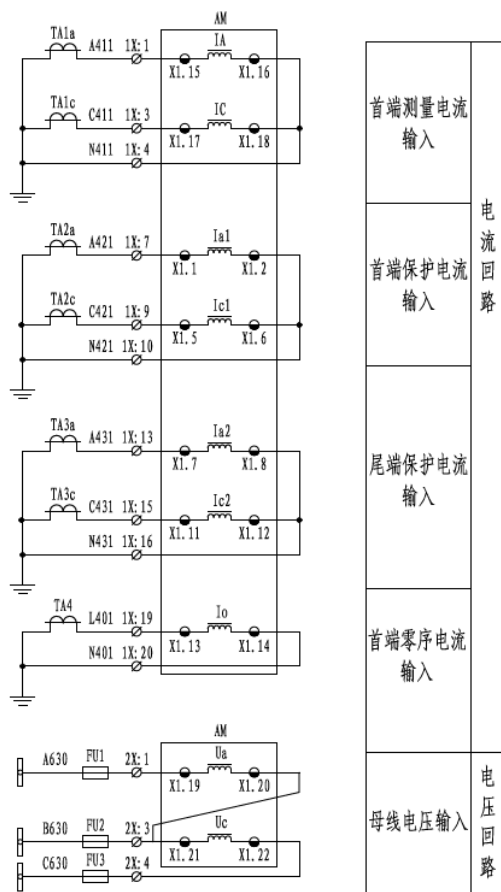
图 6.32 2PT 2CT 接线方法
