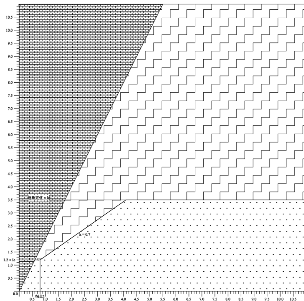
图 6.2 比例制动差动保护曲线一
