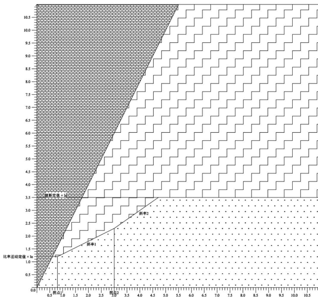
图 6.3 比例制动差动保护曲线二
