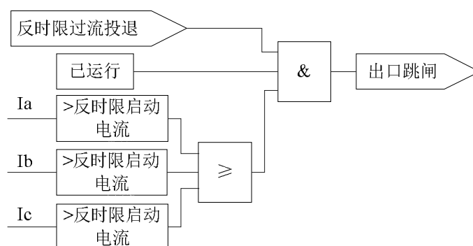
图 3.3 反时限过流保护逻辑
