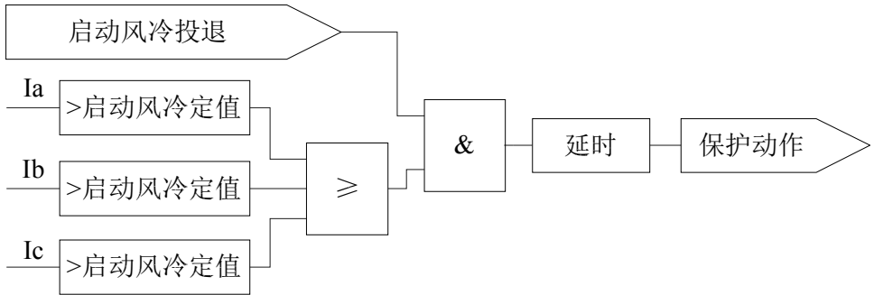
图 8.7 启动风冷保护逻辑
