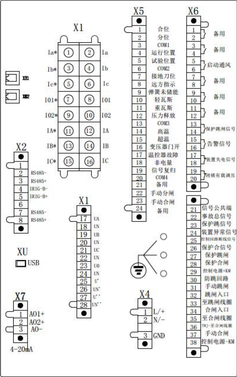
图 8.16 AM5SE-TB 电气接线图
