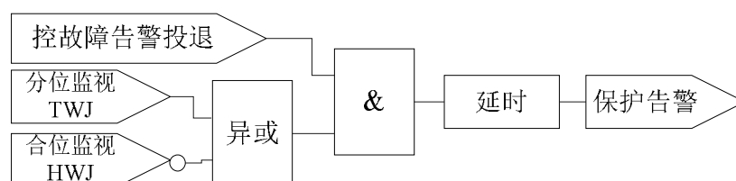
图 4.6 控制回路断线告警逻辑
