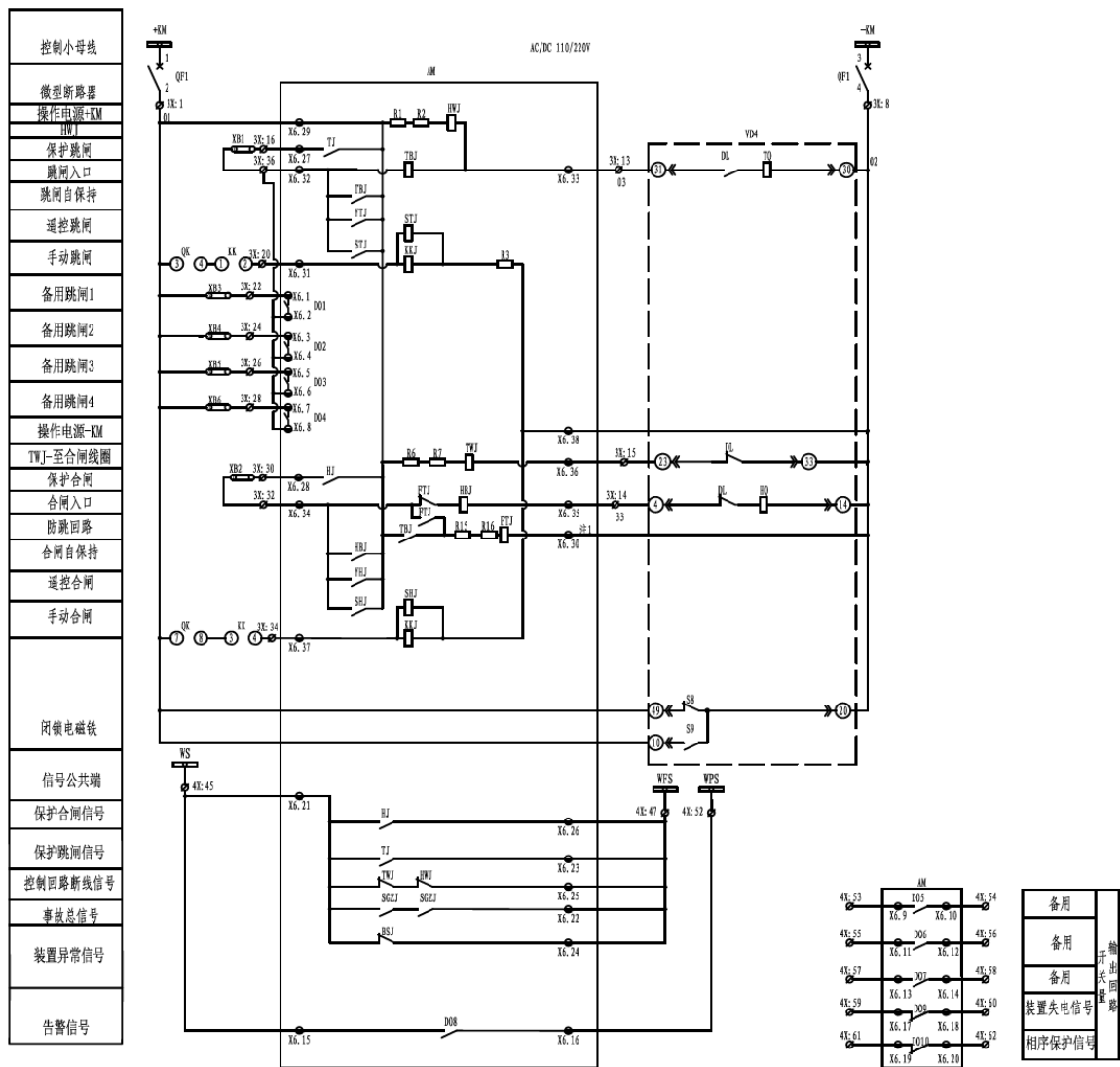
图 3.26 AM5SE-M 二次原理图（三）
