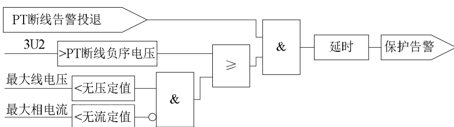
图 6.29 PT 断线告警逻辑
