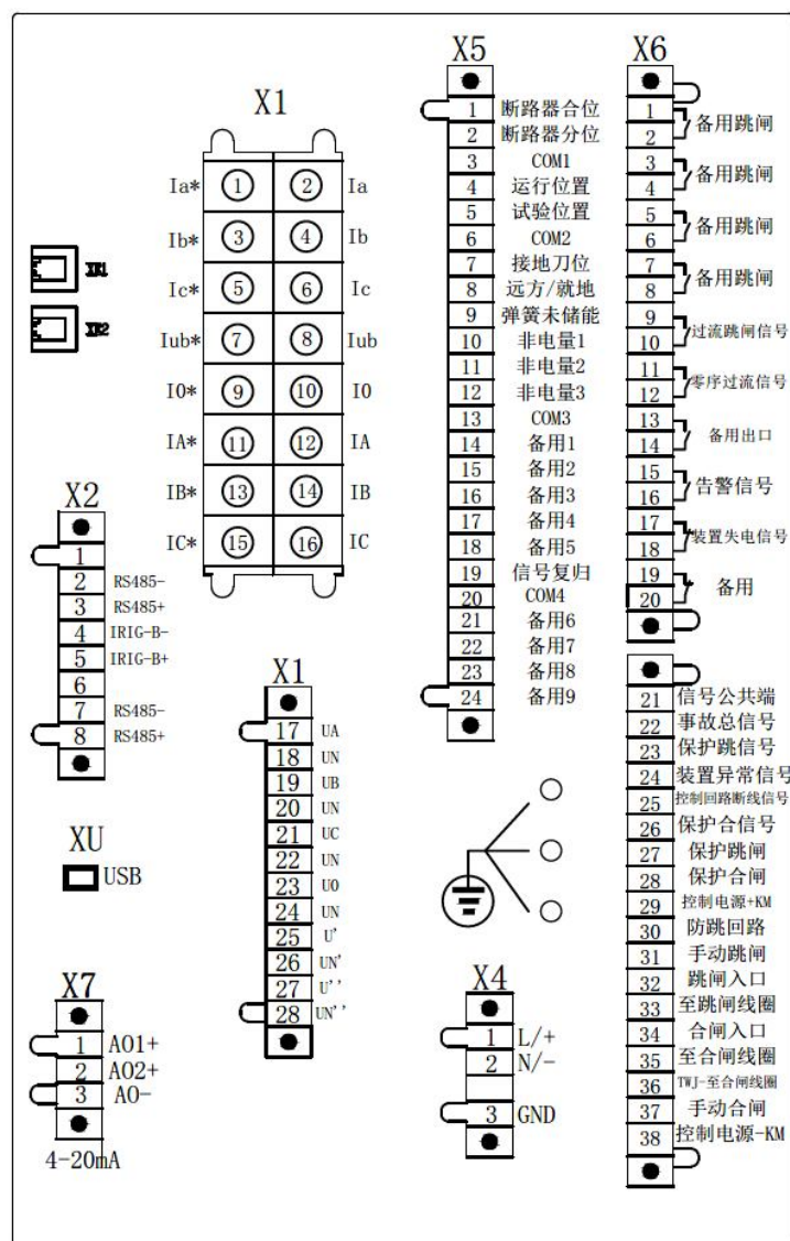
图 5.12 AM5SE-C 电气接线图
