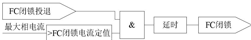
图 6.28 FC 回路配合的过流闭锁功能逻辑
