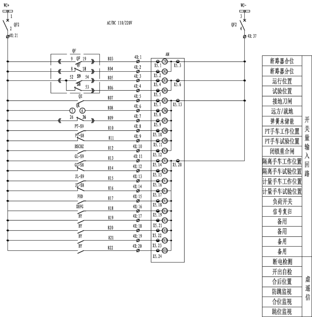
图 1.18 AM5SE-F 二次原理图（二）
