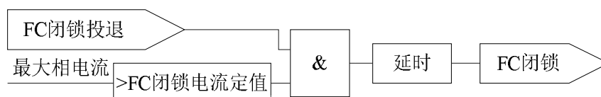
图 3.17 FC 回路配合的过流闭锁功能逻辑
