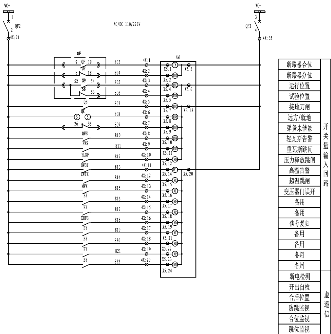
图 2.13 AM5SE-T 二次原理图（二）
