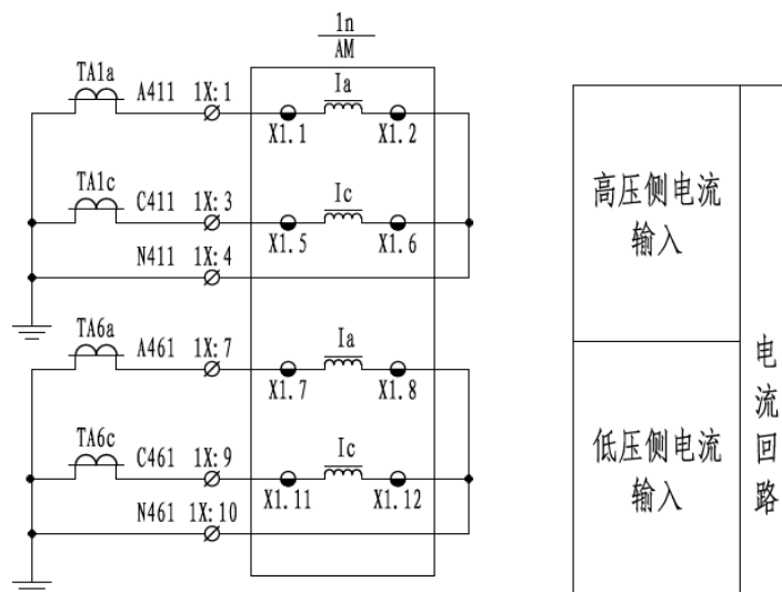
图 7.6 2CT 接线方法
