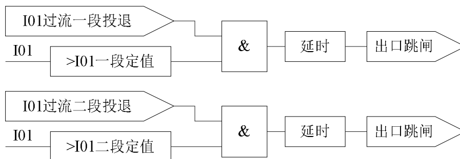
图 5.3 零序过流保护逻辑
