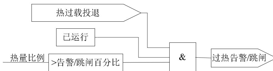
图 3.7 热过载保护逻辑
