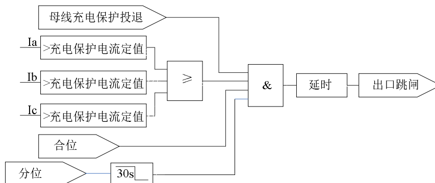
图 4.7 母线充电保护逻辑
