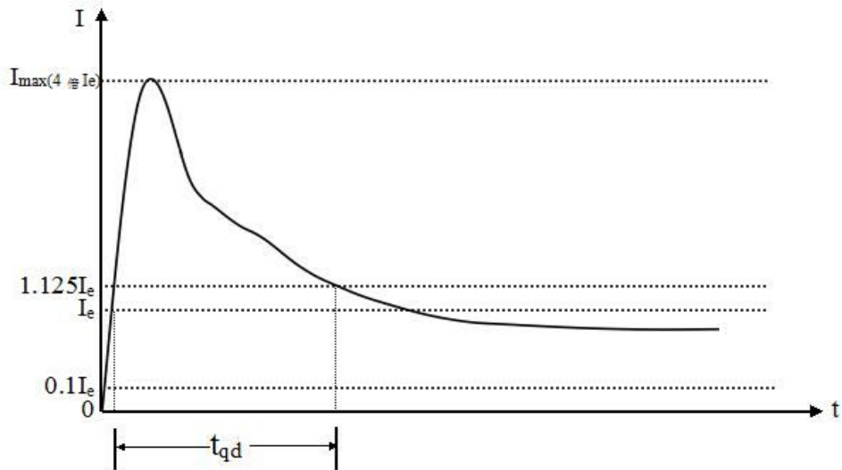
图 3.10 异步电动机启动电流特性图
