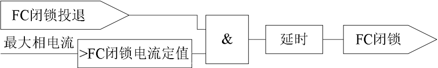
图 2.9 FC 回路配合的过流闭锁功能逻辑
