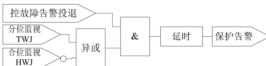
图 3.15 控制回路断线告警逻辑
