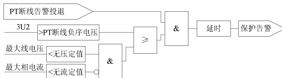
图 8.13 PT 断线告警逻辑
