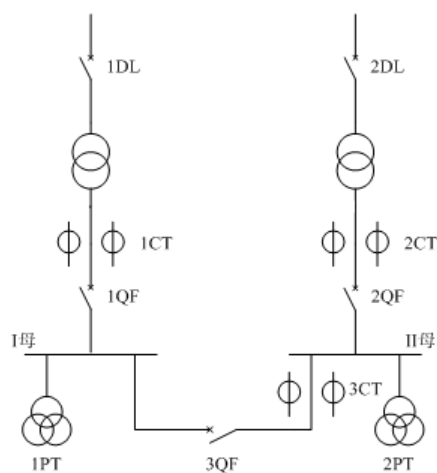
图 4.5.2 两进线一母联系统采集两段母线电压一次图
