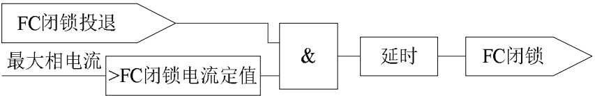
图 8.15 FC 回路配合的过流闭锁功能逻辑
