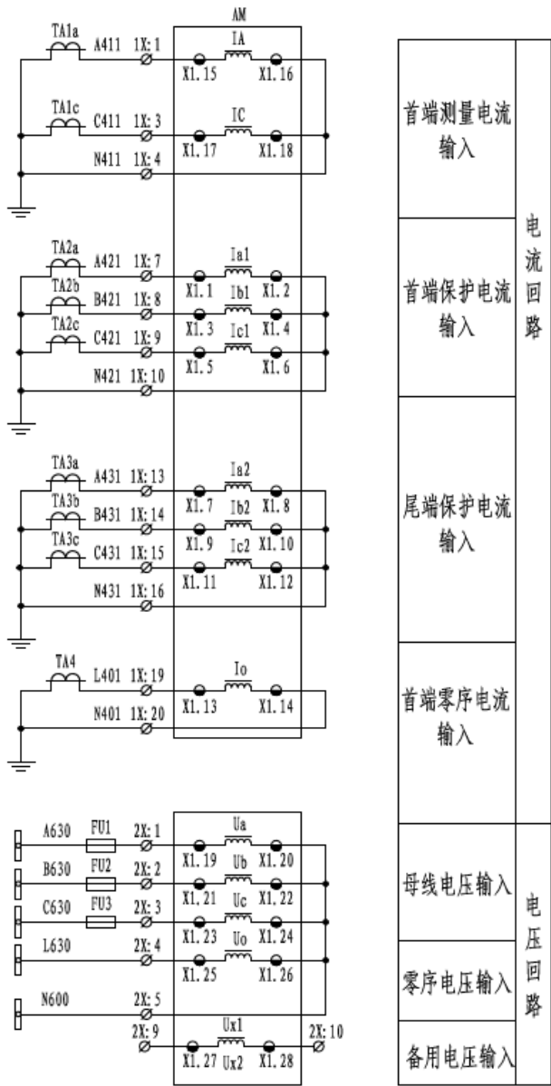
图 6.33 AM5SE-MD 二次原理图（一）
