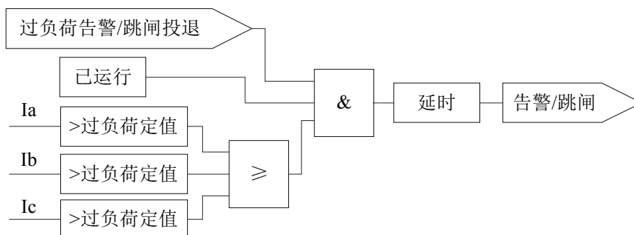
图 3.8 过负荷保护逻辑
