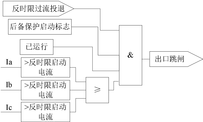
图 6.6 反时限过流保护逻辑
