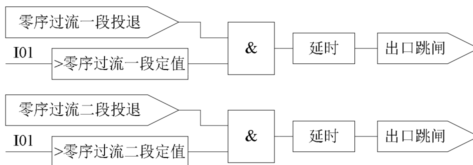
图 8.4 两段式零序过流保护逻辑
