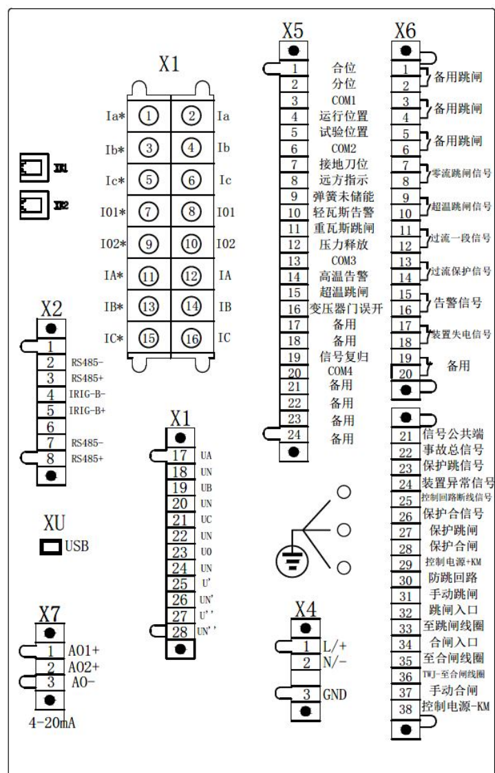
图 2.10 AM5SE-T 电气接线图
