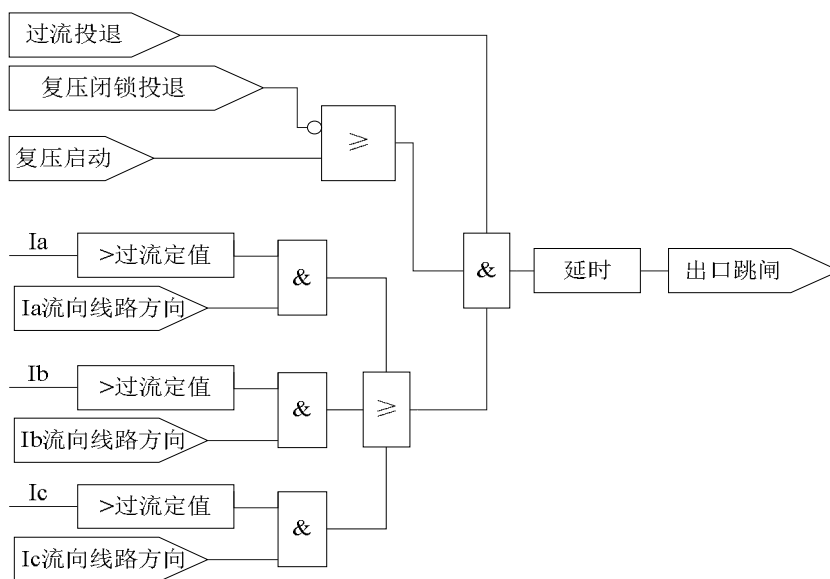
图 8.2 三段式过流保护逻辑
