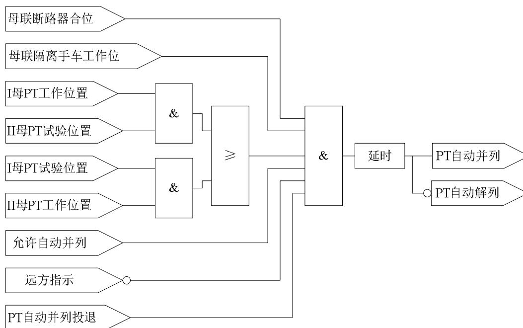
图 9.3 PT 自动并列解列逻辑
