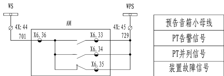
图 9.18 AM5SE-UB 二次原理图（四）
