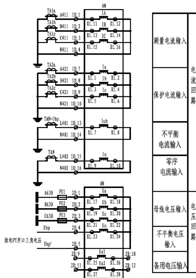
图 5.14 AM5SE-C 二次原理图（一）
