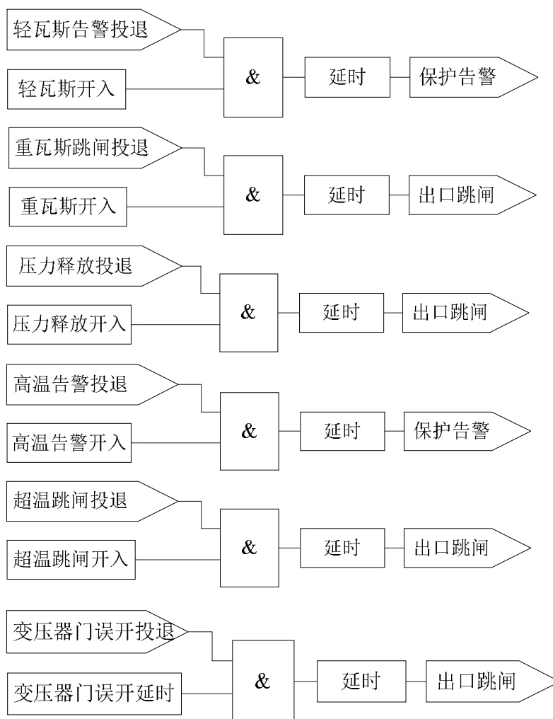
图 2.8 非电量保护逻辑
