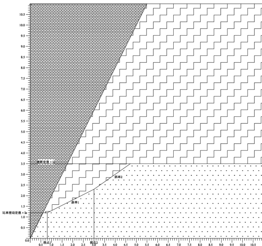
图 7.3 比例制动差动保护曲线二
