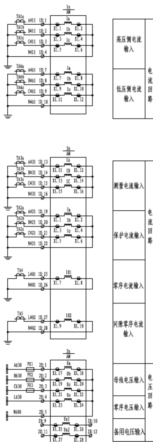
图 8.18 AM5SE-TB 二次原理图（一）
