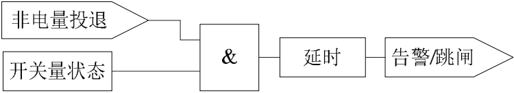
图 5.9 非电量保护逻辑
