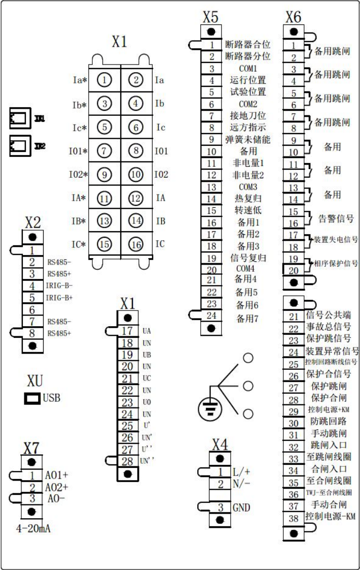
图 3.22 AM5SE-M 电气接线图
