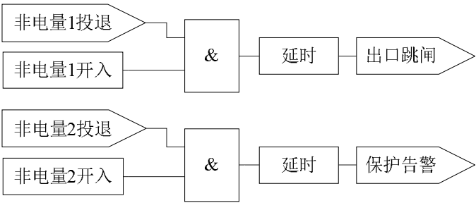
图 3.13 非电量保护逻辑
