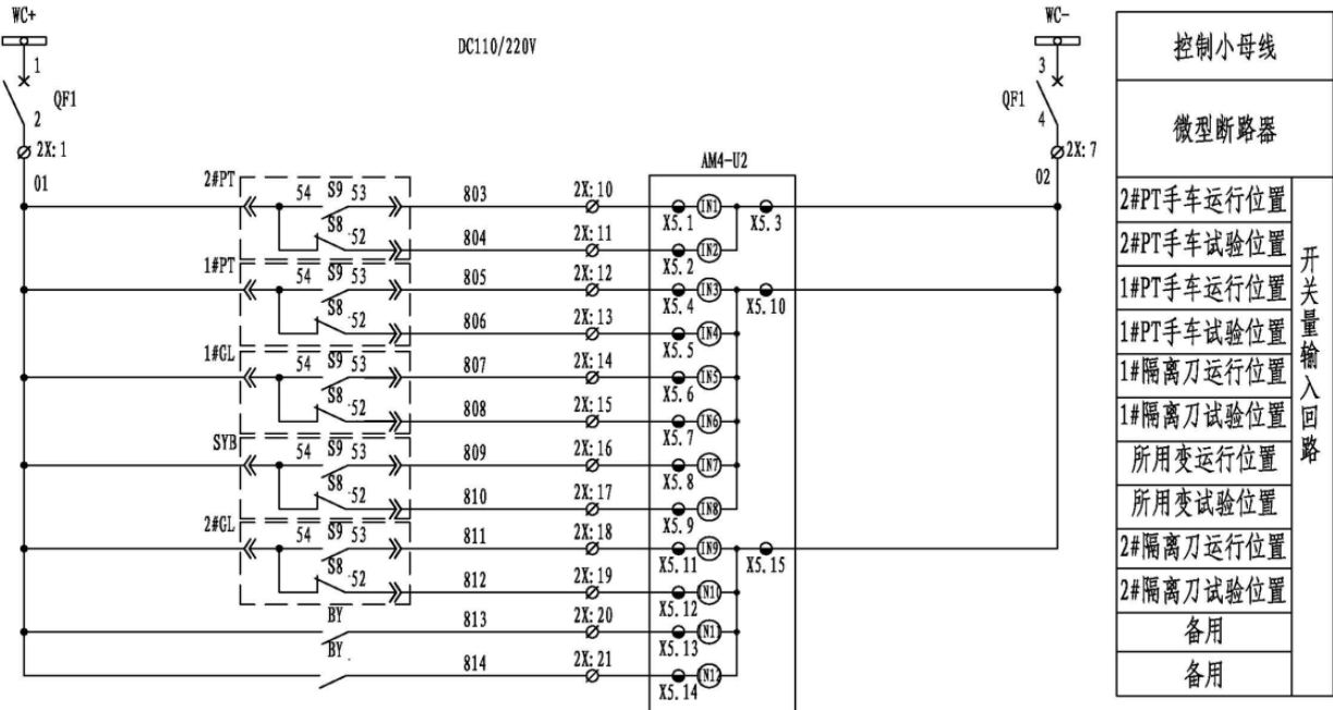
图 3.8 AM4-U2 两段母线电压保护装置二次原理图（三）
