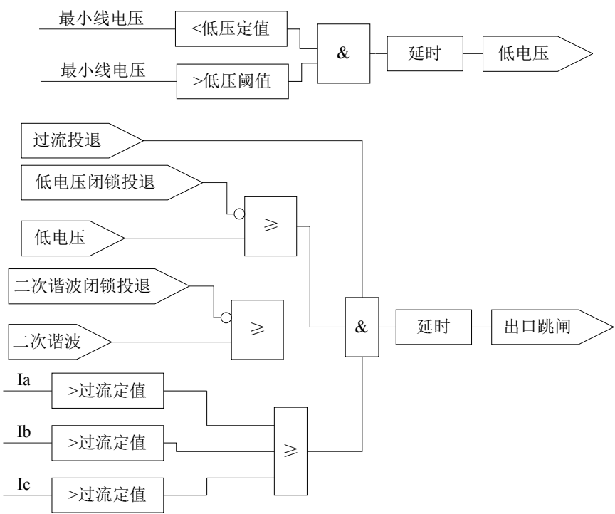
图 1.1 三段式过流保护逻辑
