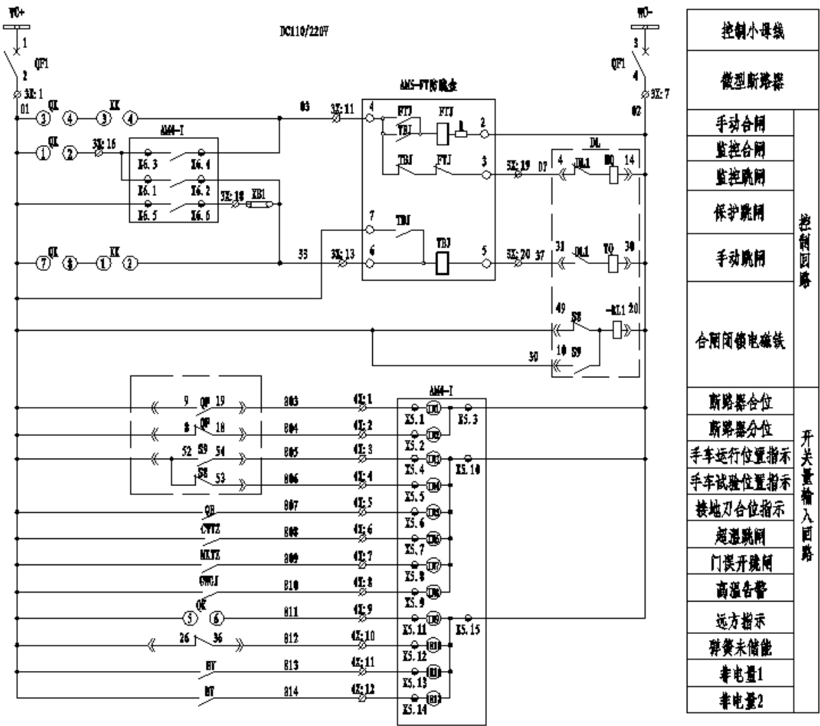
图 1.20 AM4-I 控制回路、开入回路原理图（二）
