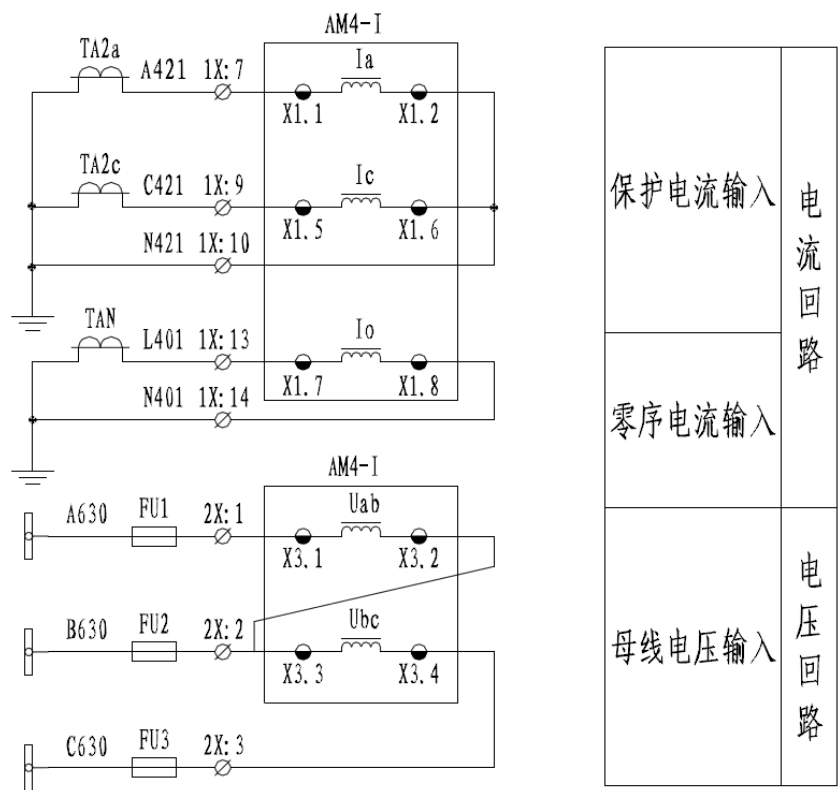
图 1.18 2PT 2CT 接线方法
