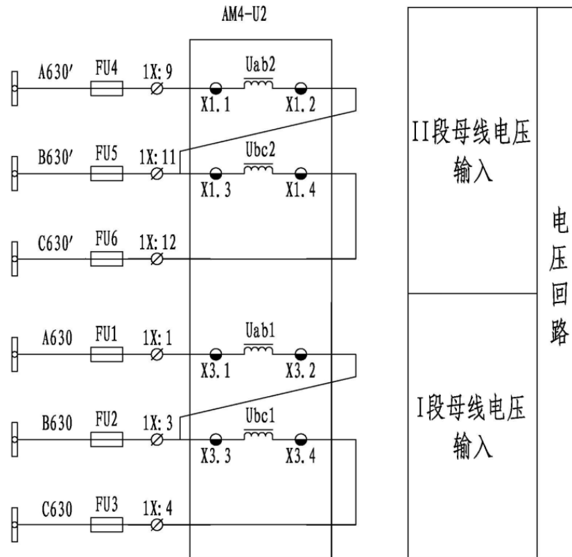
图 3.5 2PT 接线方法
