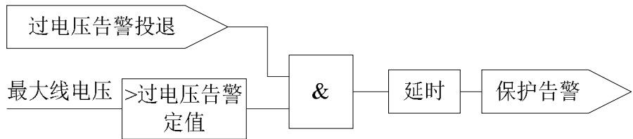
图 3.3 过电压告警逻辑
