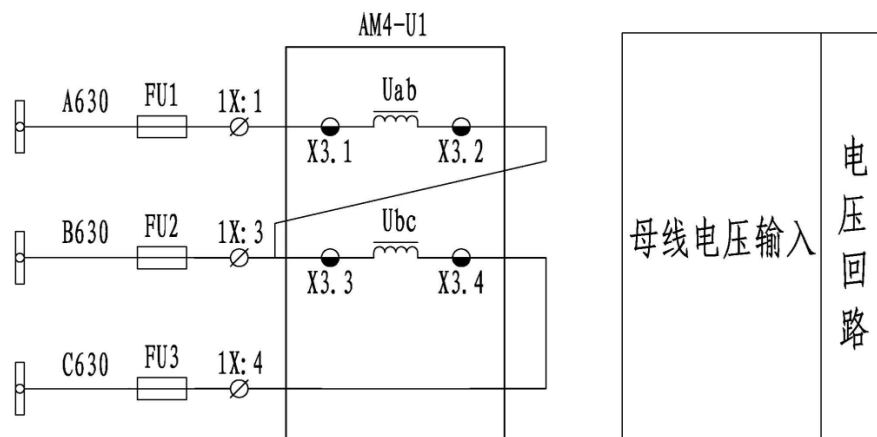
图 2.5 2PT 接线方法
