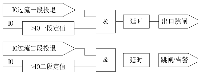
图 1.4 两段式零序 I_0 过流保护逻辑
