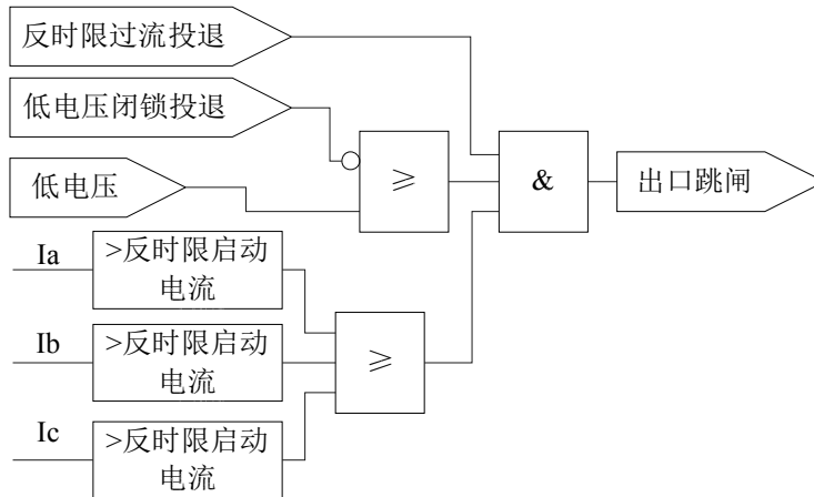
图 1.2 反时限过流保护逻辑
