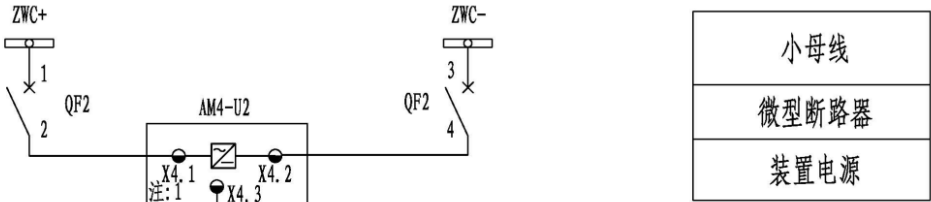
图 3.7 AM4-U2 两段母线电压保护装置二次原理图（二）
