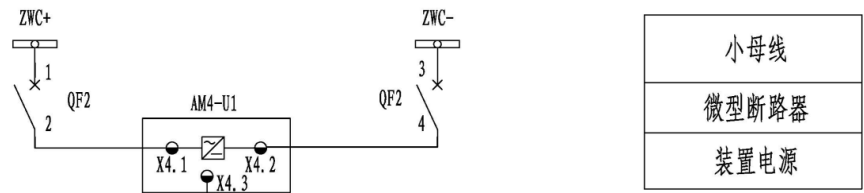
图 2.6 AM4-U1 二次原理图（一）
