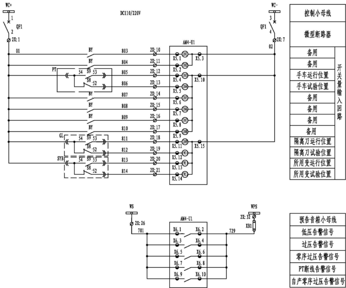
图 2.8 AM4-U1 二次原理图（三）
