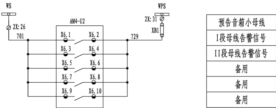
图 3.6 AM4-U2 两段母线电压保护装置二次原理图（一）
