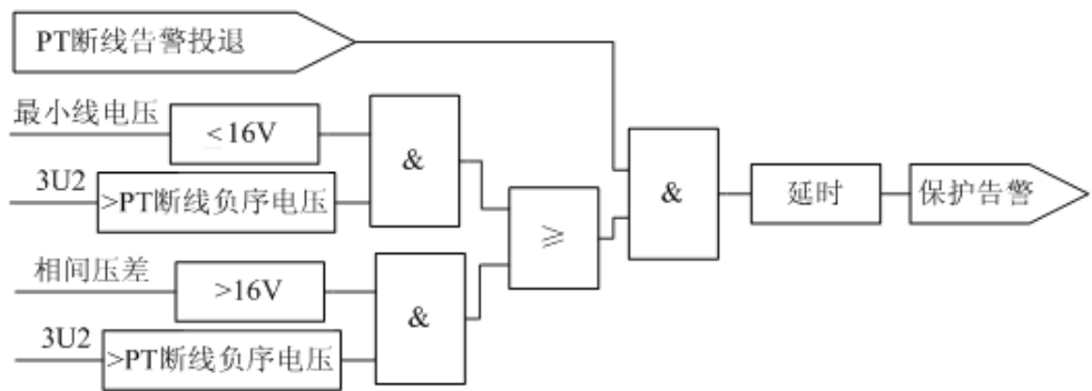
图 3.2 PT 断线告警逻辑
