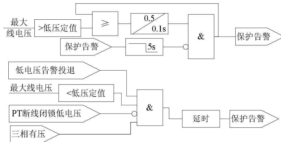
图 3.1 低电压告警逻辑
