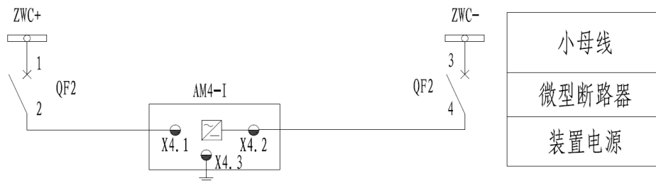
图 1.19 AM4-I 二次原理图（一）
