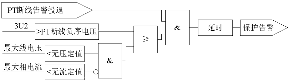
图 1.10 PT 断线告警逻辑
