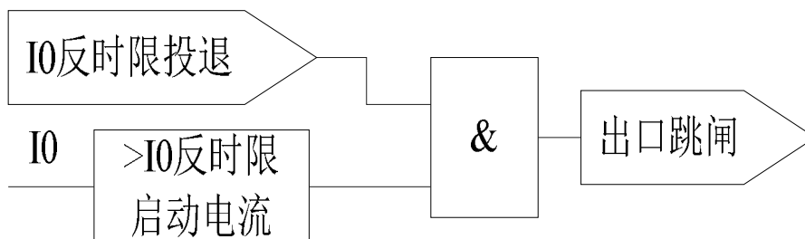
图 1.3 过负荷保护逻辑
