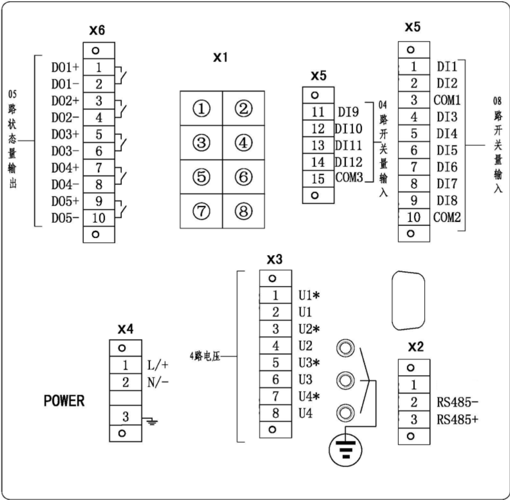
图 2.4 AM4-U1 电气接线图
