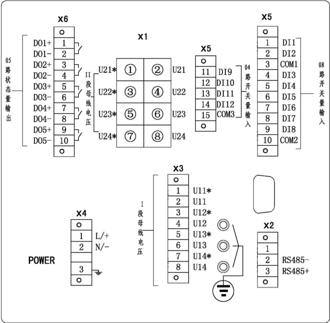
图 3.4 AM4-U2 两段母线电压保护装置电气接线图
