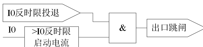
图 1.5 I_0 反时限过流保护逻辑
