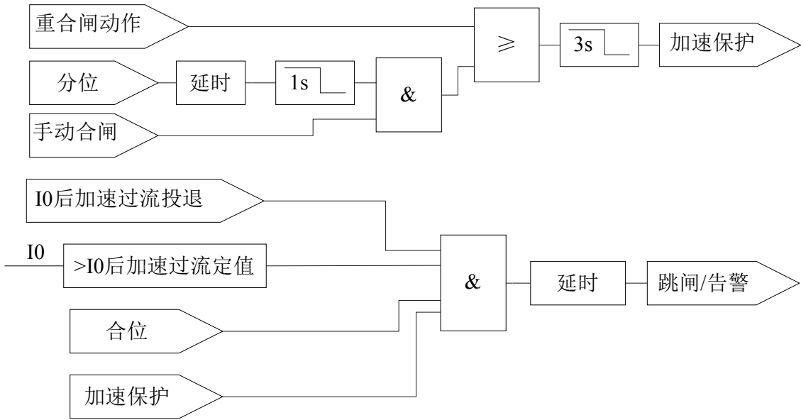
图 1.16 I0 后加速过流保护逻辑
