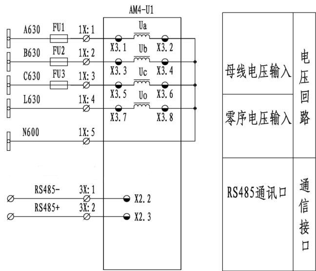
图 2.7 AM4-U1 二次原理图（二）
