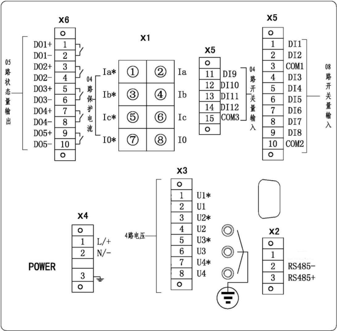
图 1.17 AM4-I 电气接线图
