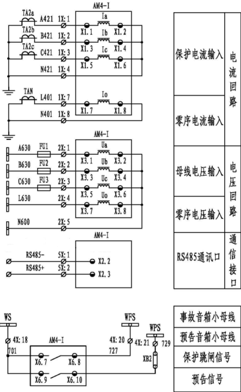
图 1.21 AM4-I 二次原理图（三）
