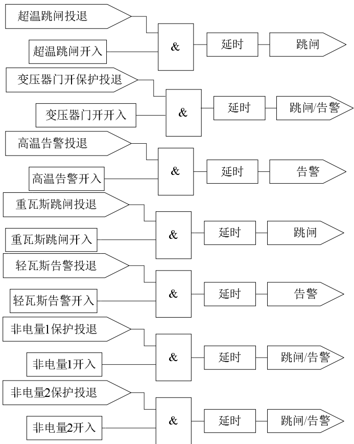
图 1.14 非电量保护逻辑
